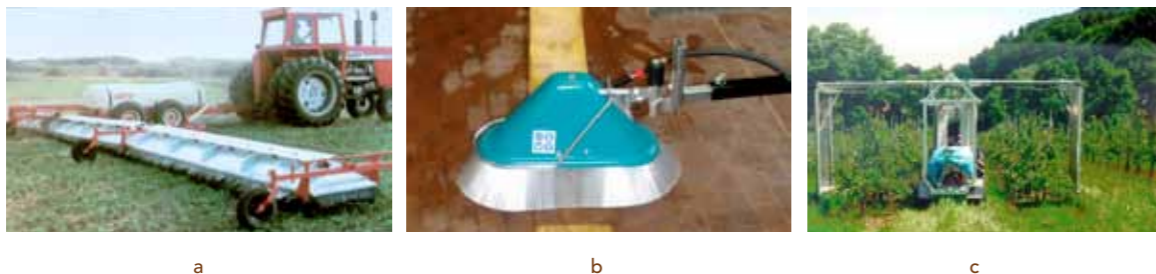
Figuur 10: Afgeschermd spuittoestel
