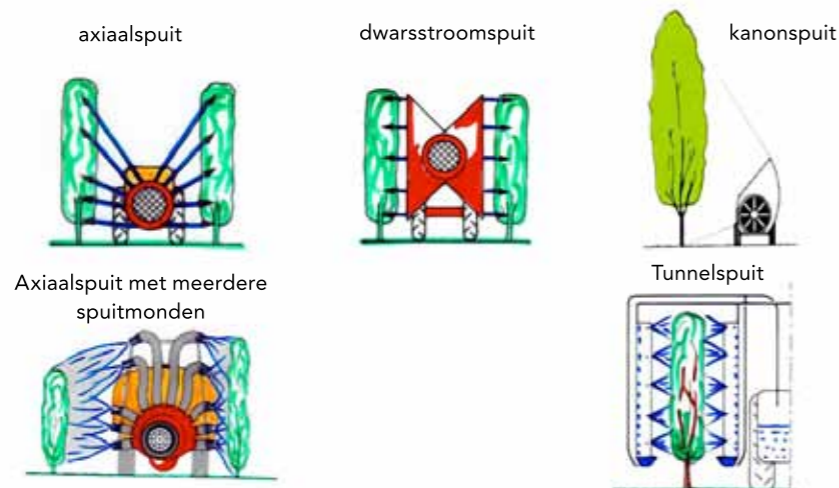
Figuur 23: Verschillende spuittoesteltypes gebruikt in boom- en wijngaarden.
